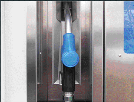
Pistolet Elaflex automatique avec clapet magnétique
